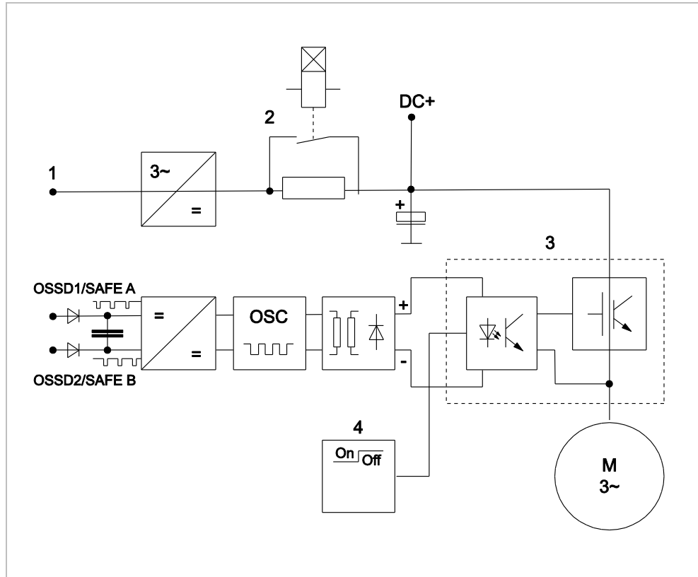
Abb. 5.6.1: Sicherheitsschaltung
