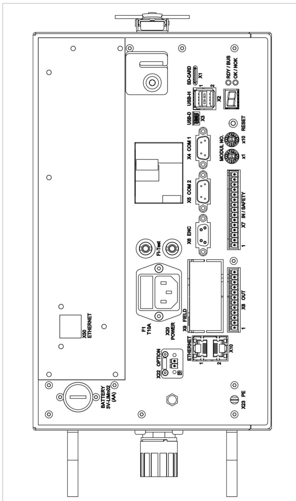
Abb. 5.3: Rückwand Steuerung
