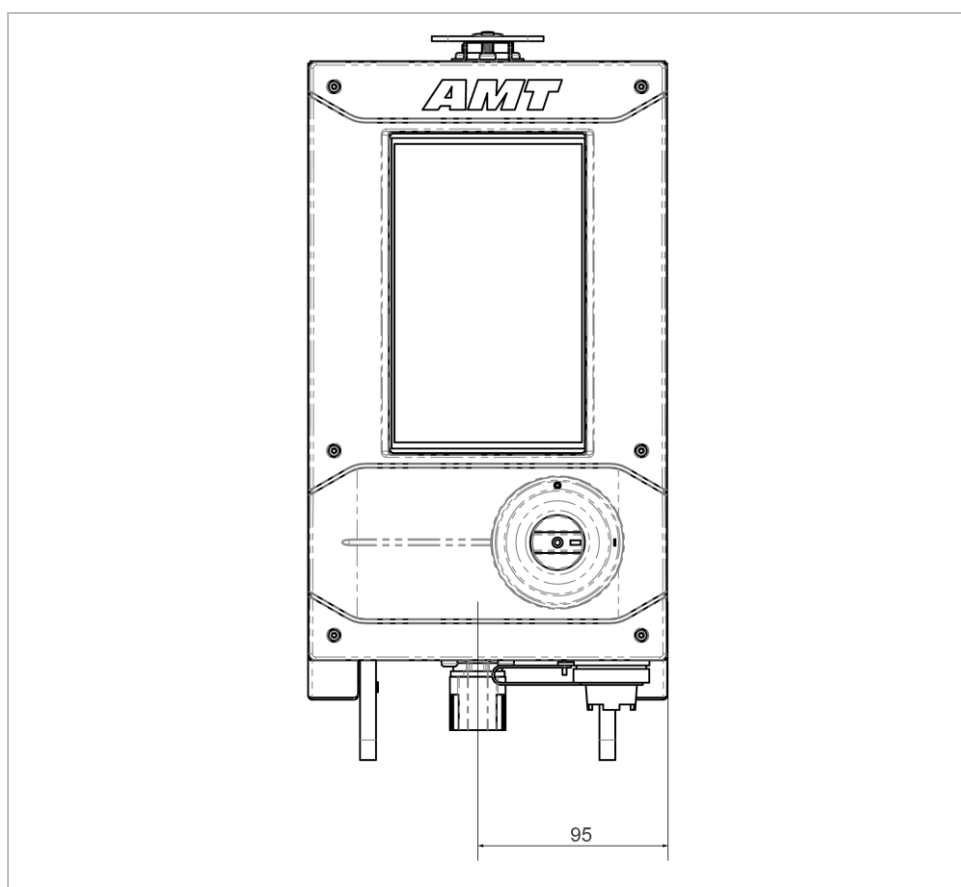
Abb. 5.4: Frontansicht
