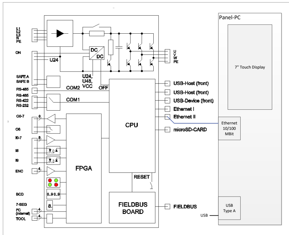
Abb. 4.4: Blockschaltbild SMX200
