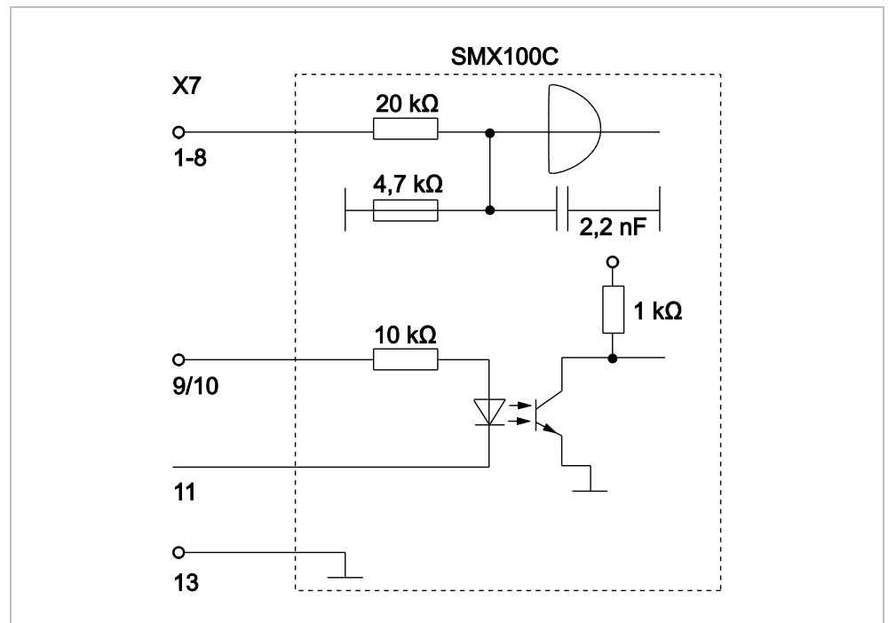
Abb. 6.5.4: X7 – Digitale Eingänge / Opto Eingänge
