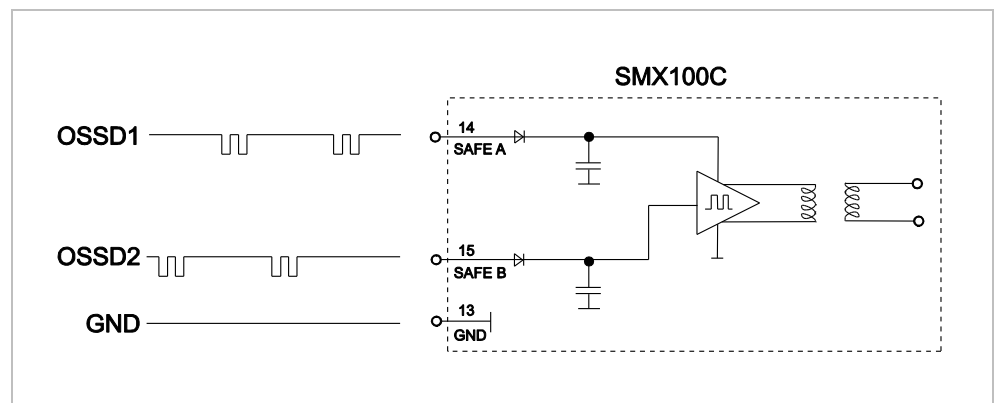
Abb. 6.5.5: Beschaltung mit OSSD
