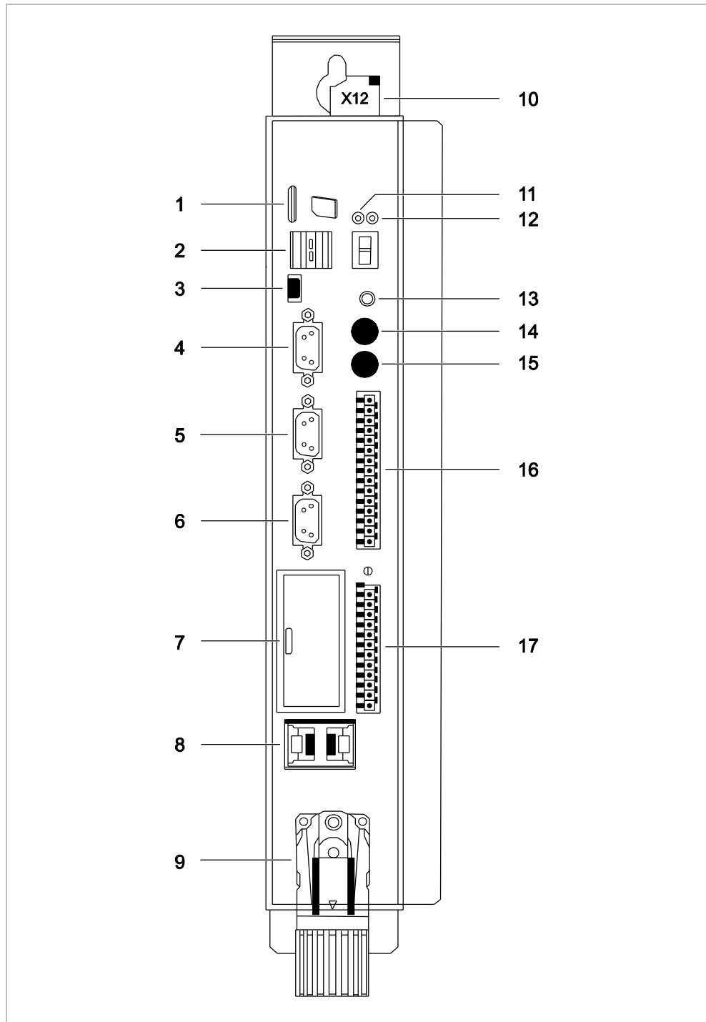
Abb. 5.4: Anschlüsse, Anzeigen und Schalter
