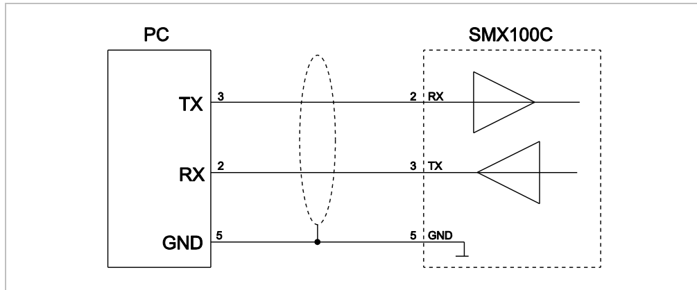
Abb. 6.5.1: COM1 – RS232
