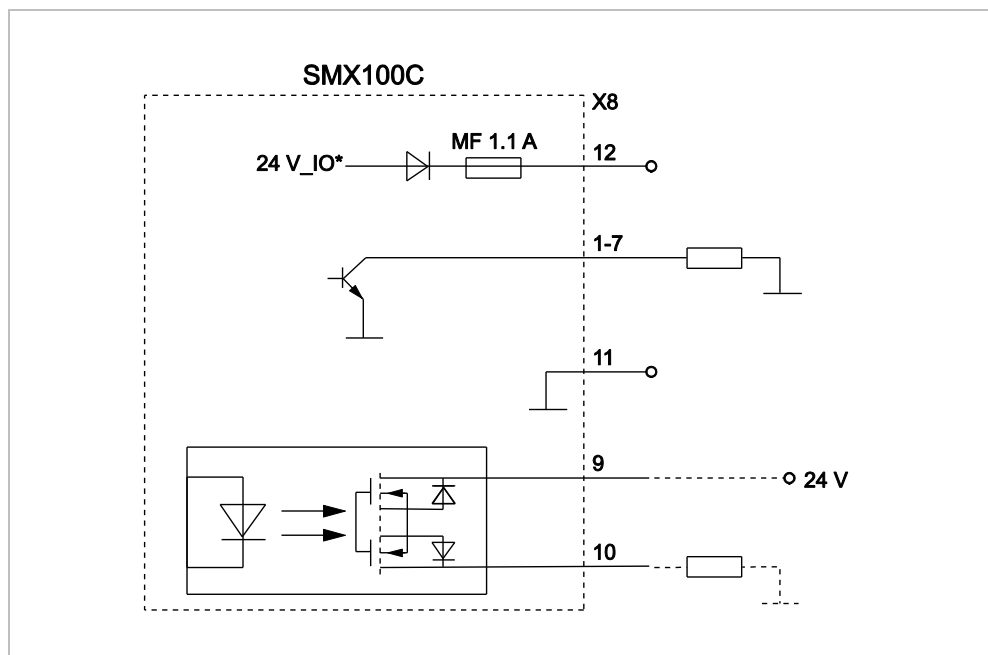
Abb. 6.5.6: X8 – Digitale Ausgänge
