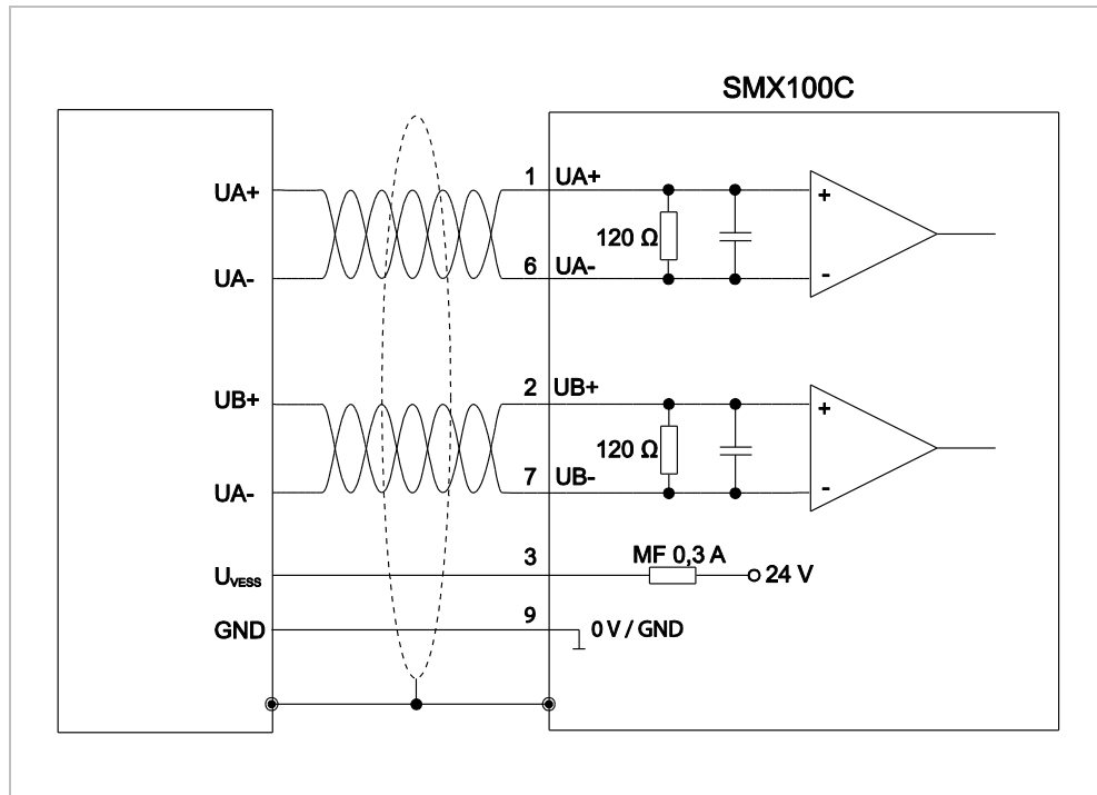
Abb. 6.5.2: X6 – Tiefenmesssystem
