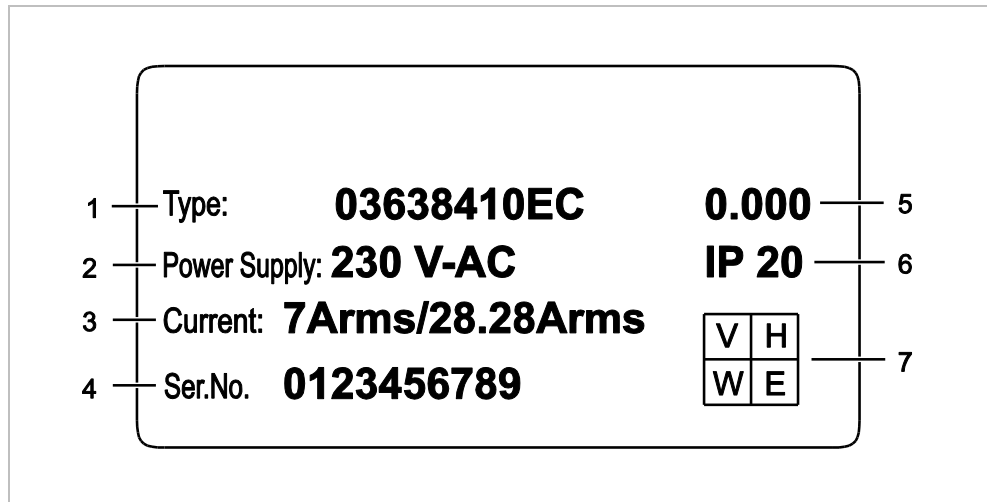
Abb. 1.9: Typenschild
