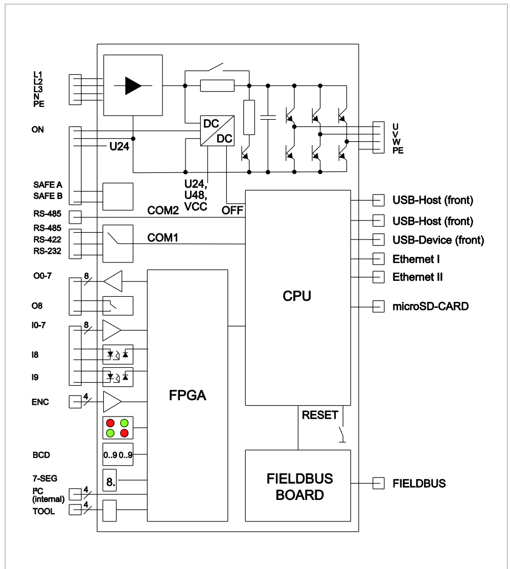
Abb. 4.3: Blockschaltbild SMX100C
