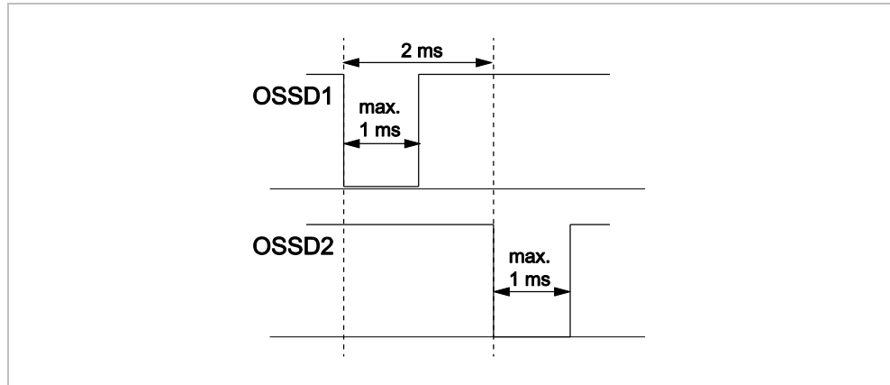
Abb. 5.6.1: OSSD Testimpulsbreite
