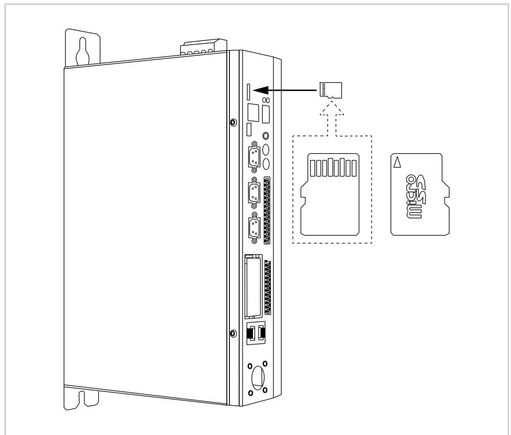
Abb. 6.4.3: Steckplatz der microSD-Card
