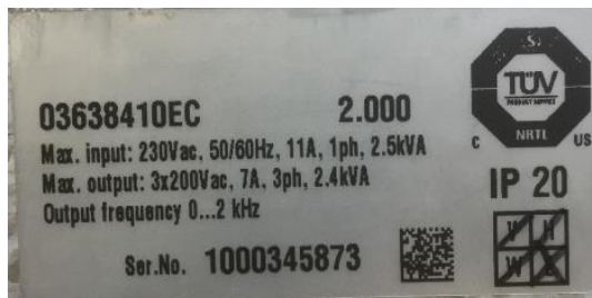
Abb. 1.9: Typenschild
