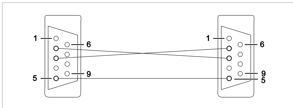
Abb. 6.5.1: Anschluss COM1 – RS232
