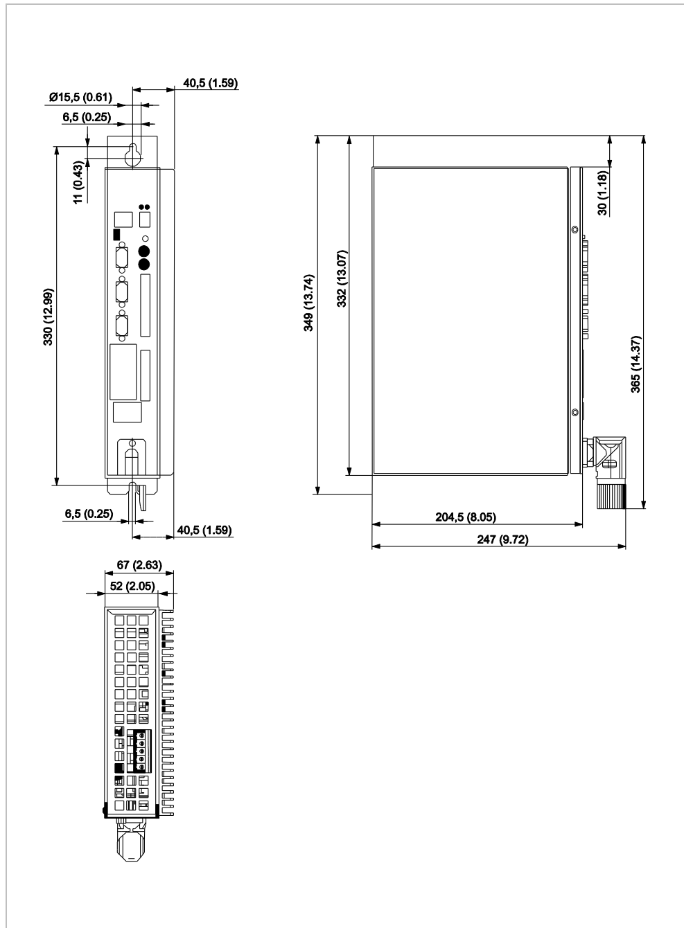
Abb. 4.2: Abmessung SMX100C. Alle Angaben in mm (inch).
