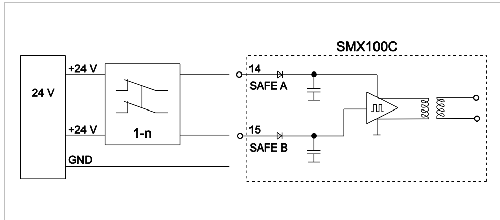
Abb. 6.5.5: Beschaltung ohne OSSD
